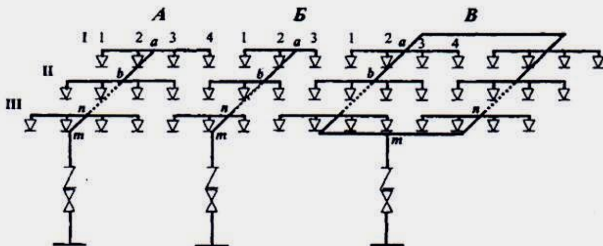
Рис. 1 Схемы распределительной сети спринклерной или дренчерной АУП:
